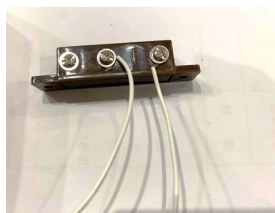
C共用點 + NO常開點
